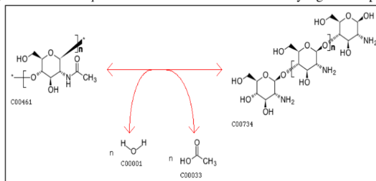
Gambar 2. Struktur Kitosan
