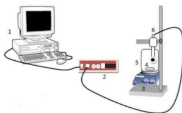
Gambar 1. Rangkaian alat sensor QCM (Kurniawan dan Madurani., 2015; Kurniawan et al. , 2017; Nugroho dan Kurniawan., 2015; Nurramdaniyah et al. , 2017)
