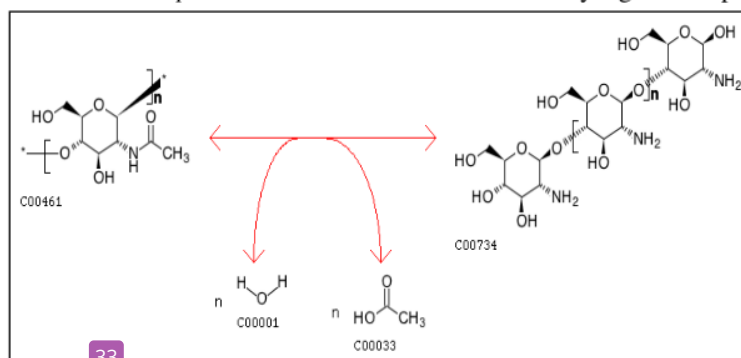
Gambar 2. Struktur Kitosan
