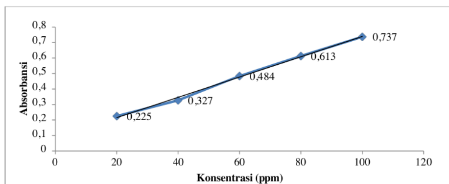
Gambar 2. Kurva Baku Standar Kuarsetin
