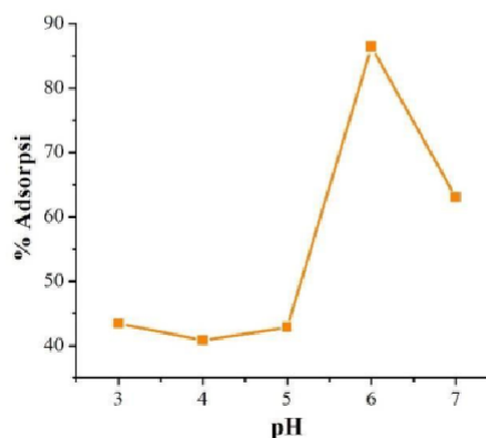
Gambar 2. Grafik hasil adsorpsi logam Fe terhadap variasi pH larutan
