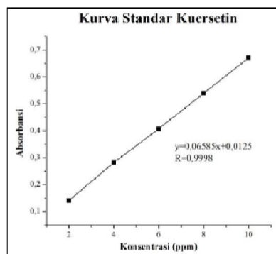
Gambar 1 Kurva standar kuersetin pada panjang gelombang 434,2 nm
