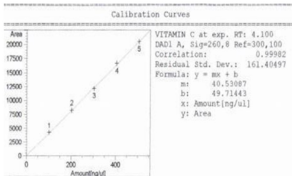
Gambar 1. Kurva Kalibrasi Standar Vitamin C
